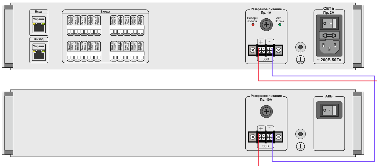
Рис. 2.1 Подключение устройства к БРП-36/07
