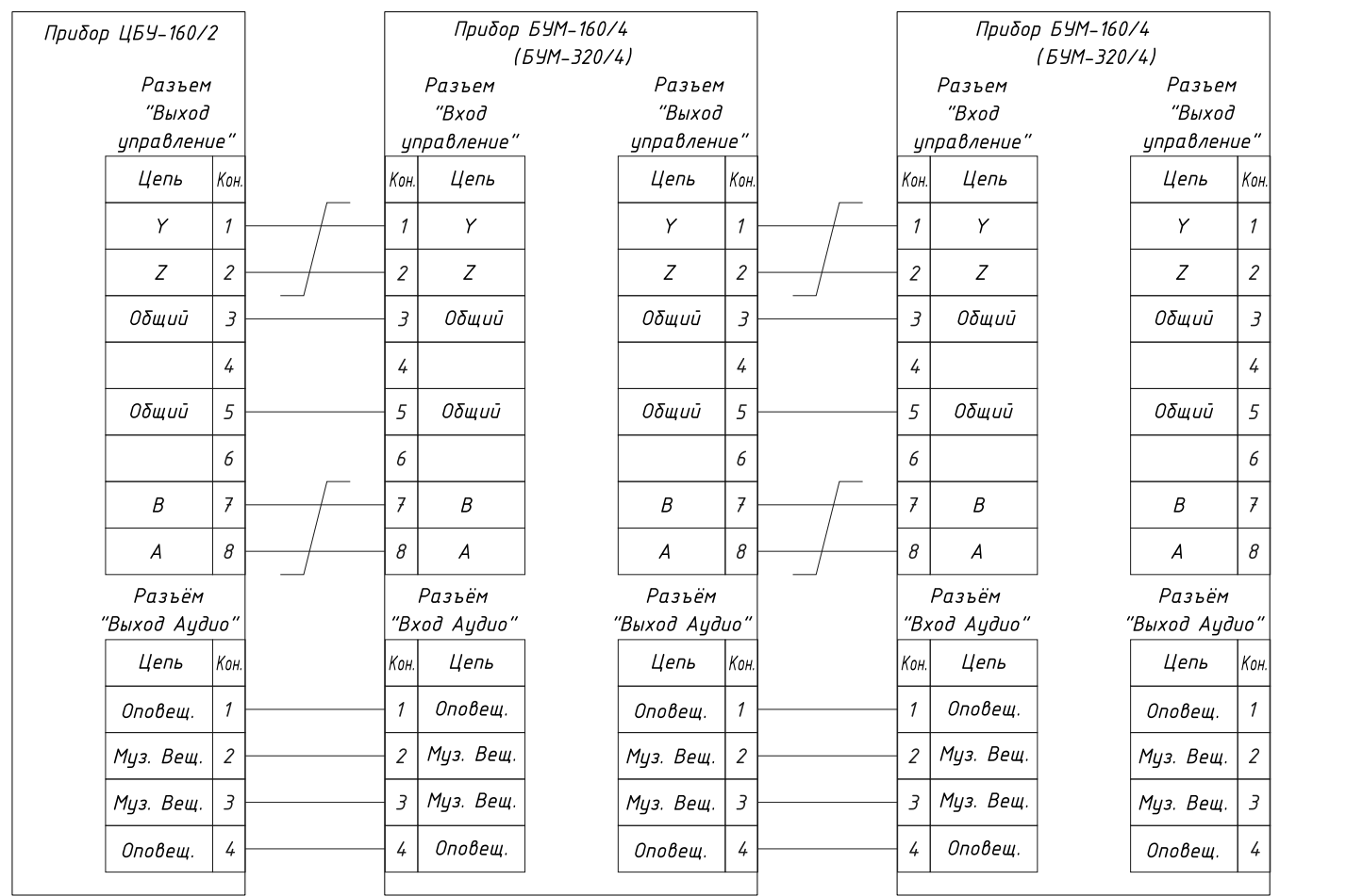
Рис. 1.4. Пример подключения устройства к блоку ЦБУ-160/2
